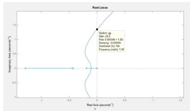
Fig.6. Root Locus
