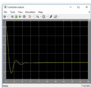
Fig.12.1. Controller Output
